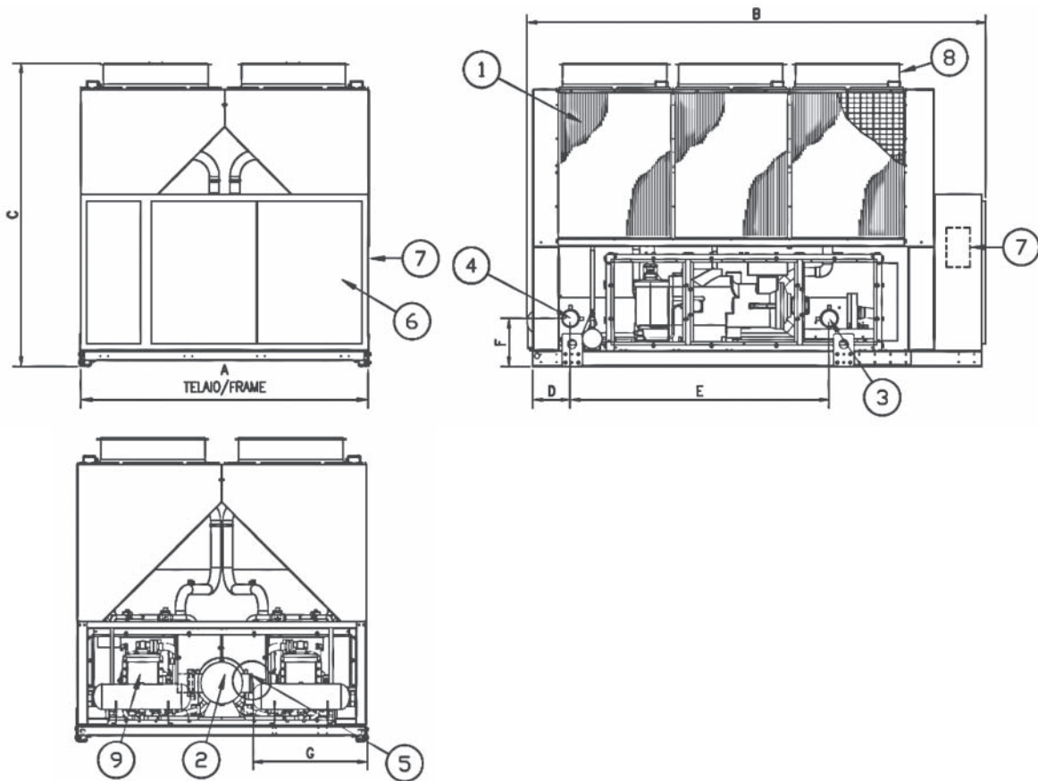
Dimensions EWYD~BZ
