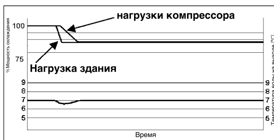
Неустойчивость EWLТ с плавным регулированием производительности
