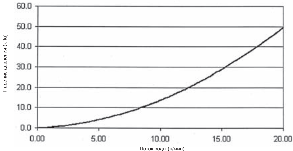
Падение давления в FWF02B7TV1B
