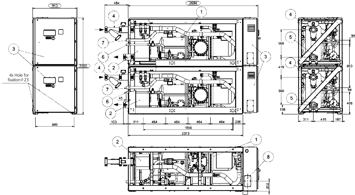
EWLD-J-SS / 2 Circuits
