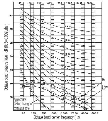
FXZQ20,25M9
