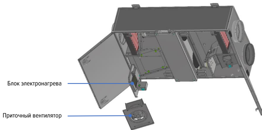
Рис. 30. Обслуживание электронагревателя
