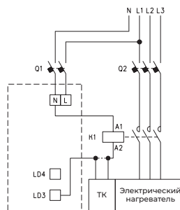
Рис. 19. Схема подключения трехфазного электронагревателя
