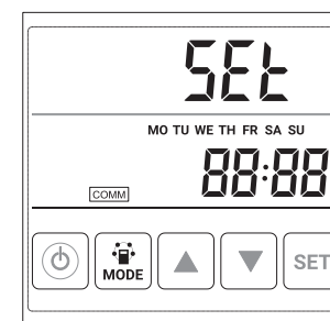
Рис. 45. Установка дня недели.
