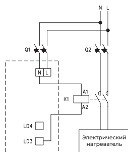
Рис. 17. Схема подключения однофазного электронагревателя
