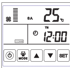
Рис. 27. Температура SA (приточного воздуха)
