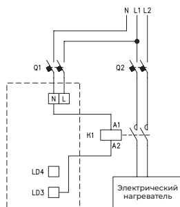
Рис. 18. Схема подключения двухфазного электронагревателя
