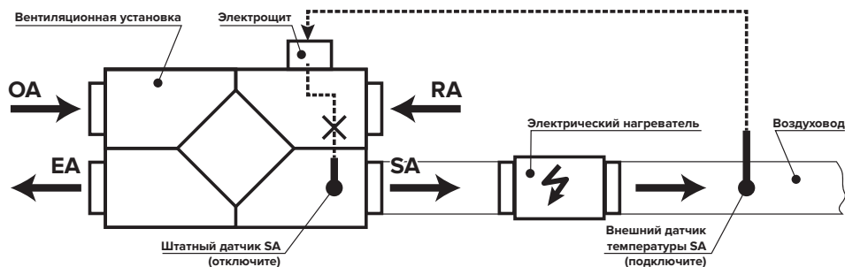
Рис. 11. Подключение внешнего датчика температуры SA
