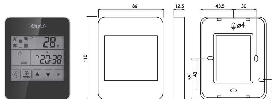
Рис. 22. Пульт управления SRC-TS
