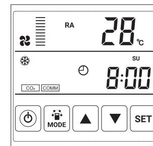
Рис. 63. Индикация режима размораживания.
