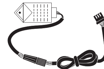
Рис. 32. Датчик влажности в комплекте с кабелем 5 м.
