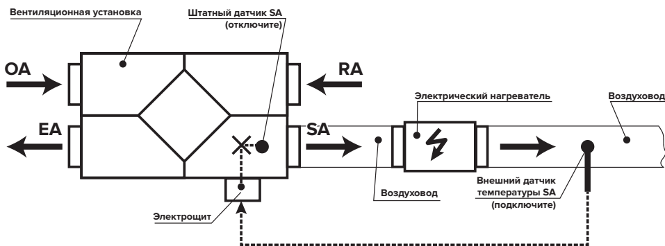
Рис. 13. Подключение внешнего датчика температуры SA
