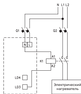
Рис. 20. Схема подключения двухфазного электронагревателя
