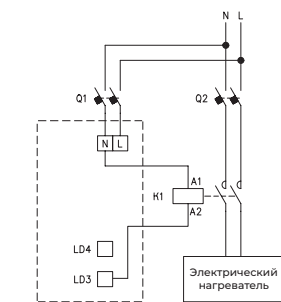
Рис. 19. Схема подключения однофазного электронагревателя
