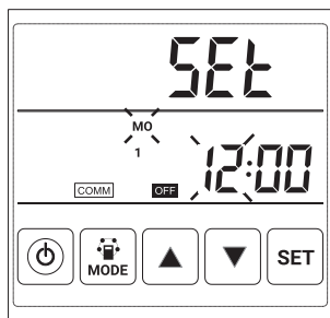
Рис. 63. Установка часов таймера выключения.
