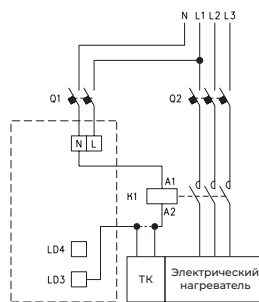
Рис. 21. Схема подключения трехфазного электронагревателя
