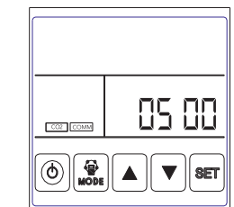
Рис. 32. Концентрация CO 2
