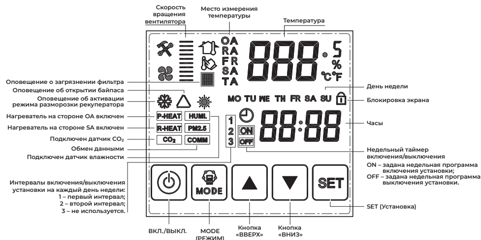
Рис. 24. Пользовательский интерфейс
