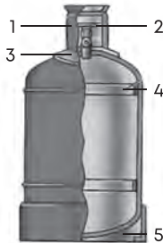
Рис. 3. Баллон
