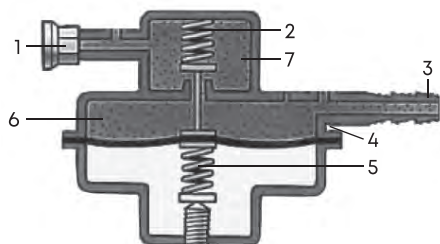
Рис. 4. Редуктор
