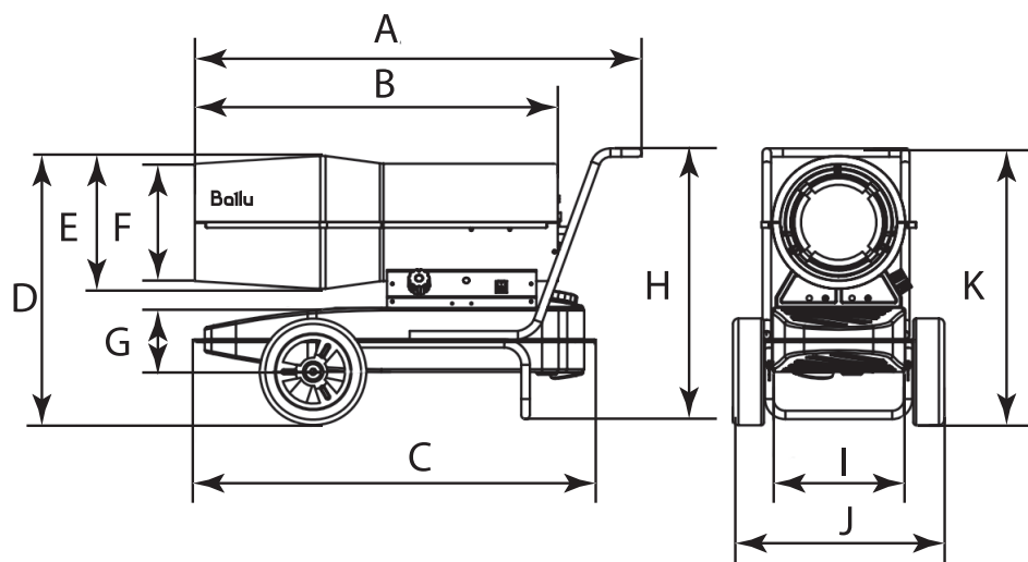
Рис. 4. Размеры прибора BHDP-30, BHDP-50.
