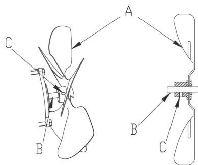
Рис. 18. Крепление крыльчатки.
