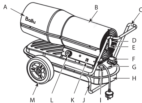
Рис. 2. Для моделей BNDP-30, BNDP-50.
