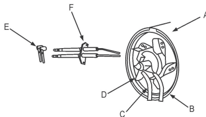
Рис. 11. Горелка.
