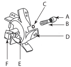
Рис. 14. Сборка горелки ВНДР-50.
