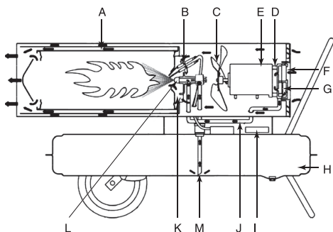
Рис. 9. Устройство защиты.
