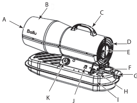
Рис. 1. Для моделей BNDP-10, BNDP-20.
