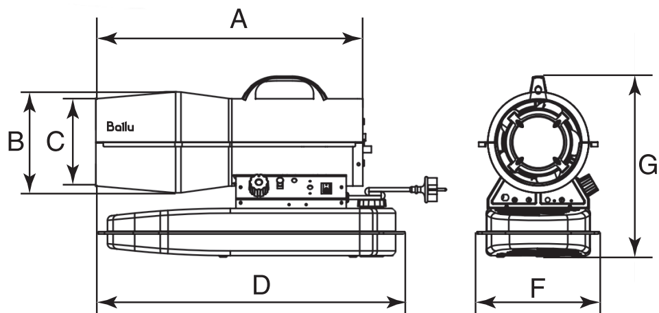
Рис. 3. Размеры прибора BHDP-10, BHDP-20.
