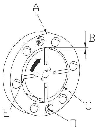
Рис. 17. Устройство насоса.
