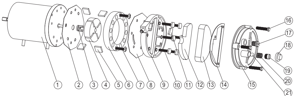
Рис. 16. Воздушный насос (компрессор).
