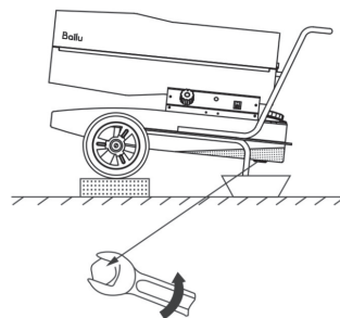
Рис. 10. Опорожнение топливного бака для ВНДР-30, ВНДР-50.
