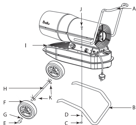
Рис. 5. Установка колес и каркаса.
