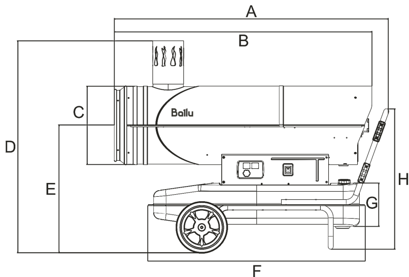
Рис. 2. Размеры.
