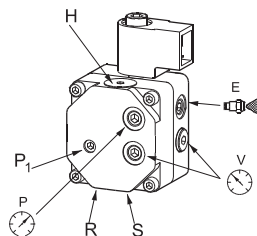
Рис. 12. Топливный насос.
