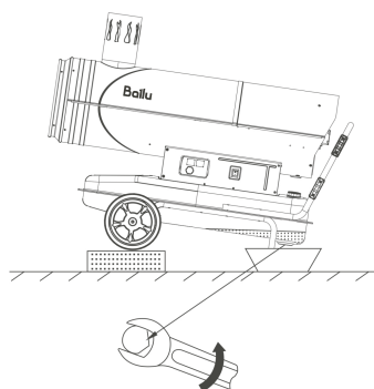
Рис. 10. Опорожнение топливного бака.
