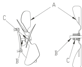
Рис. 13. Крепление крыльчатки.
