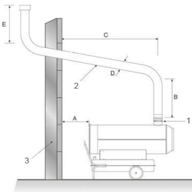
Рис. 14. Подключение отвода продуктов горения.
