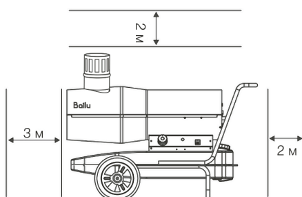
Рис. 6. Безопасные дистанции.
