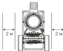
Рис. 7. Безопасные дистанции.
