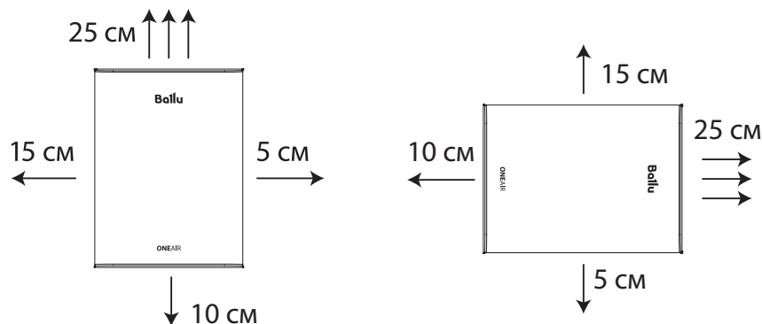
Вертикальное расположение с выпуском воздуха вверх
