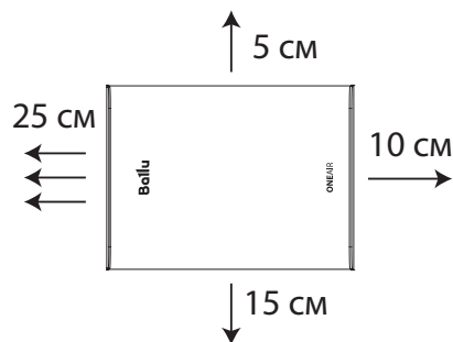
Горизонтальное расположение с выпуском воздуха слева
