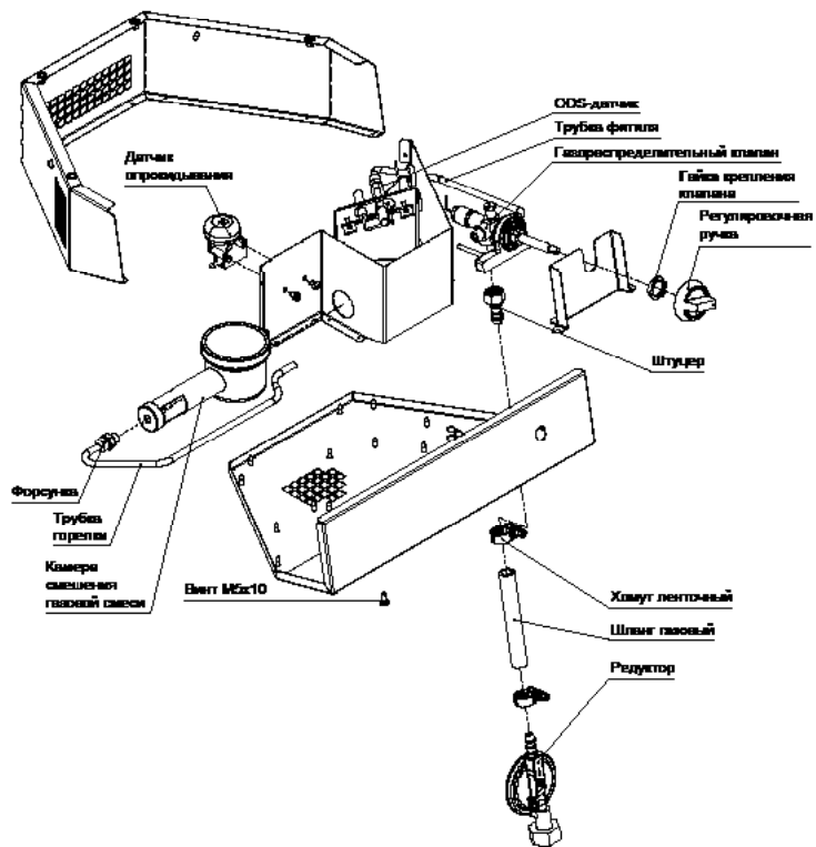
Рис. 3. Устройство блока управления (приборного отсека)
