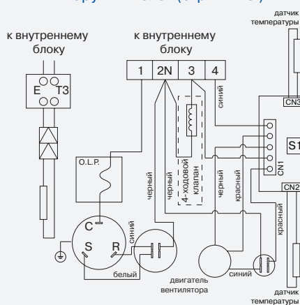
наружный блок (стр. 72-73)
