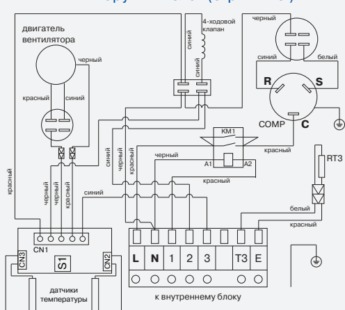
наружный блок (стр. 74-75)
