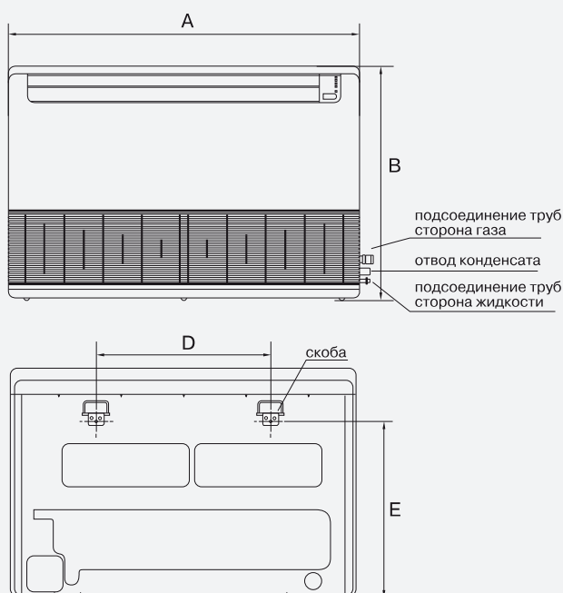
установка на стену
